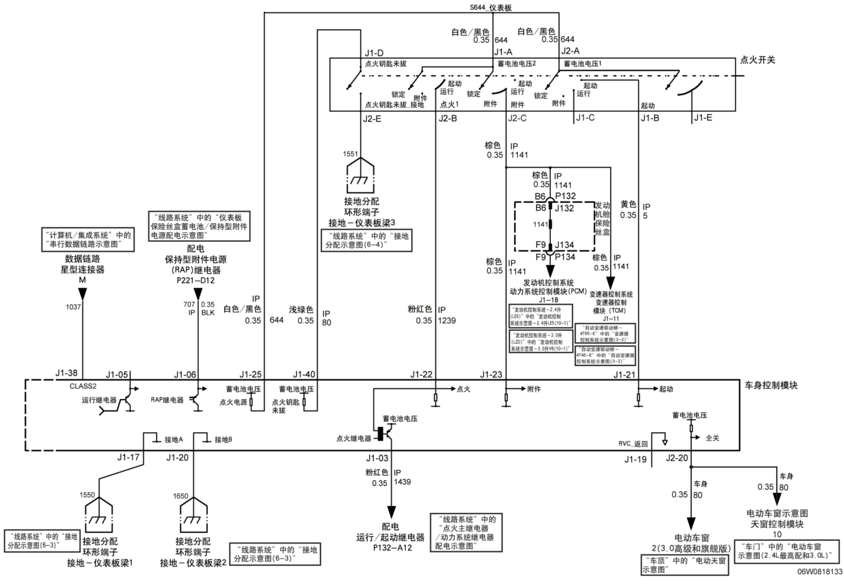
点火开关配电示意图
